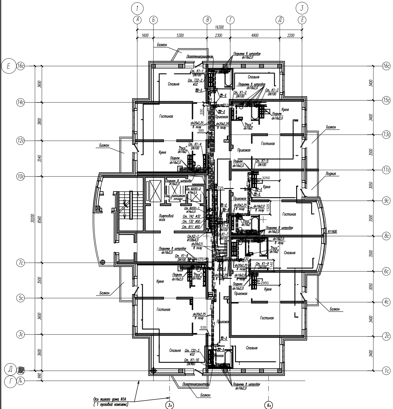
Размещение квартирных водомерных узлов в общей нише III зона (14-21 этажи)
