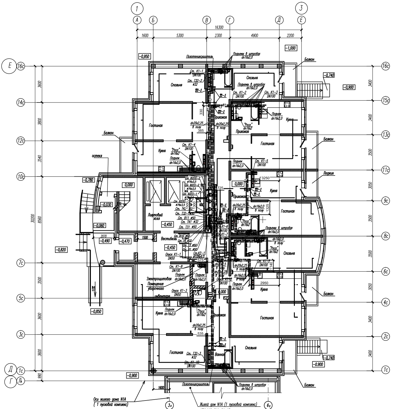
Размещение квартирных водомерных узлов в общей нише 1 зона (1-4 этажи)
