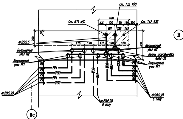
Размещение квартирных водомерных узлов в общей нише III зона (14-21 этажи)
