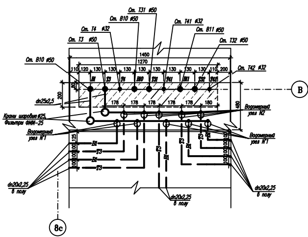
Размещение квартирных водомерных узлов в общей нише 1 зона (1-4 этажи)
